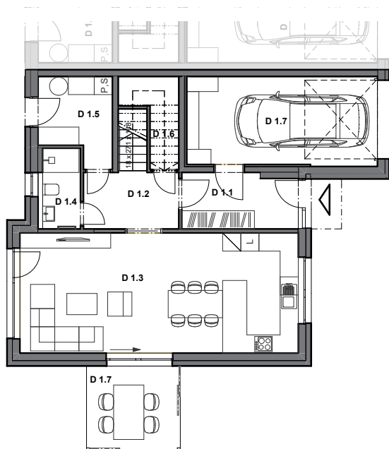
PŮDORYS 1. NP
